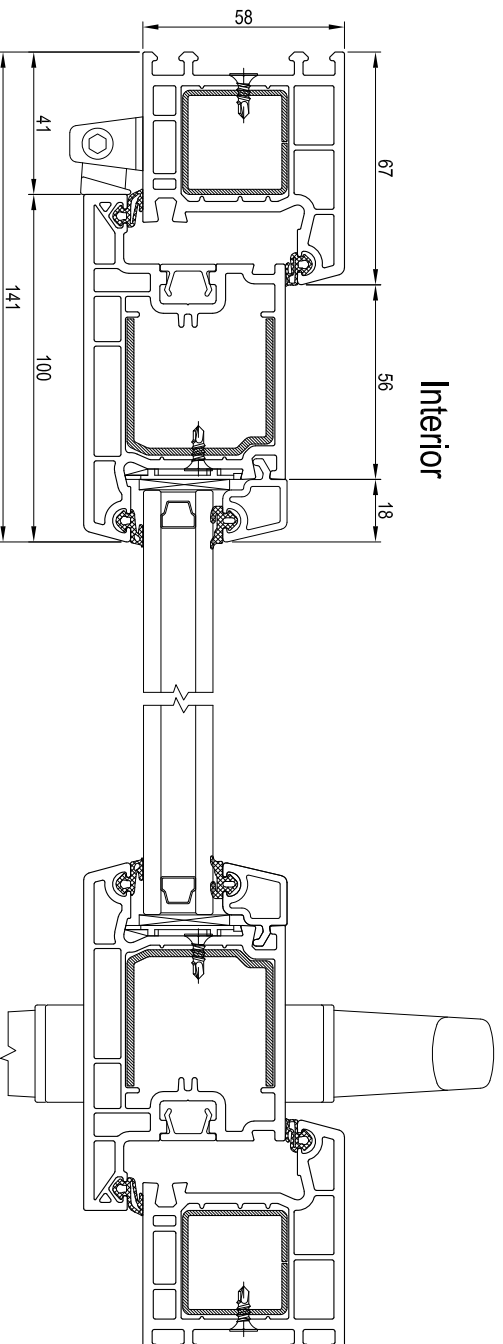
CORTE B-B
