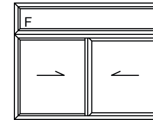
Corredera 2 hojas+fijo
