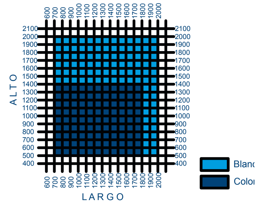
Corredera 2 hojas+fijo
