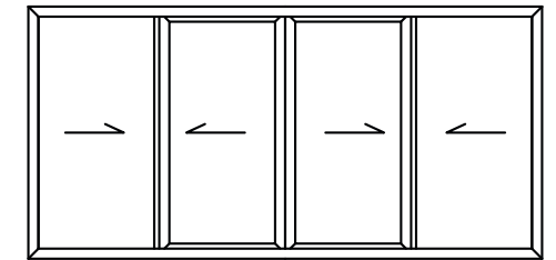
Corredera 4 hojas
