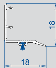
Traslazo 105.372
